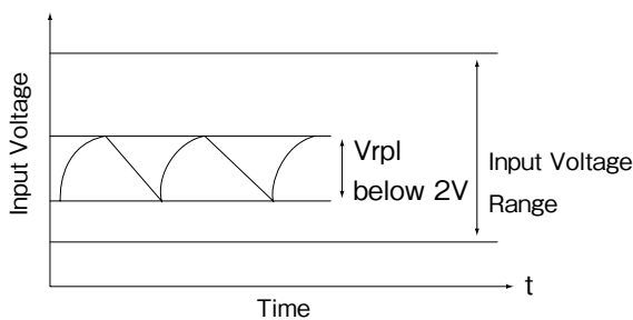
Fig.1-1 Input Ripple Voltage
