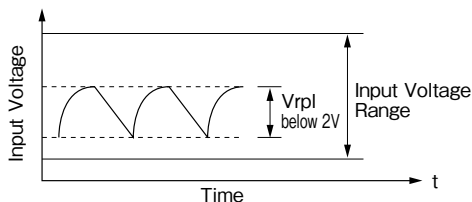
Fig.1-1 Input Ripple Voltage
