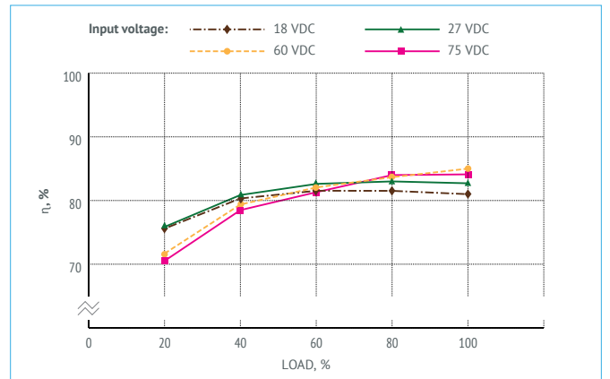
Figure 6 (d). Efficiency of MDVx50-1W27.
