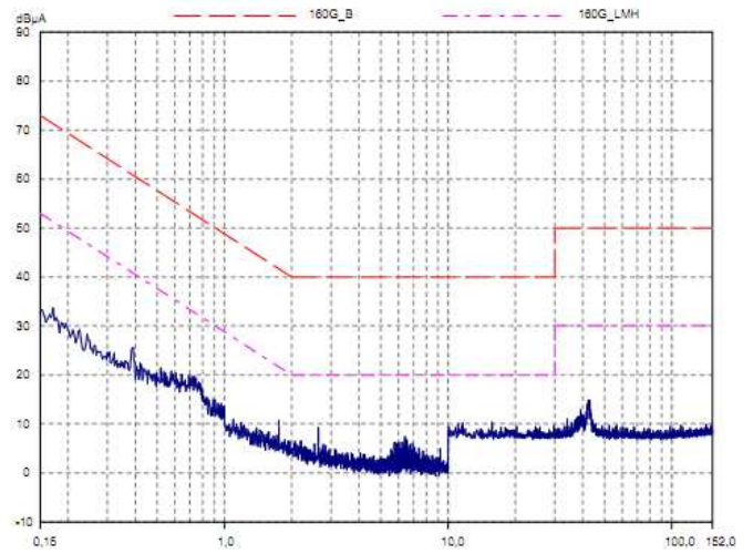
D0-160G : MGDS-75-O-J with FGDS-10A-50V
